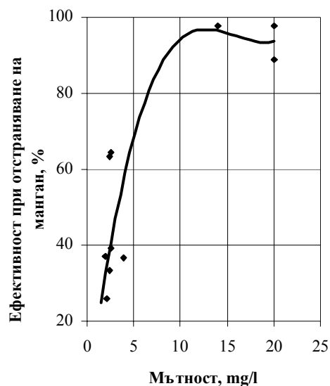
Фиг. 4.2.12. Влияние на мътноста спрямо ефективността за отстраняване на мангана от водата на яз.Искър с помощта на CFS
